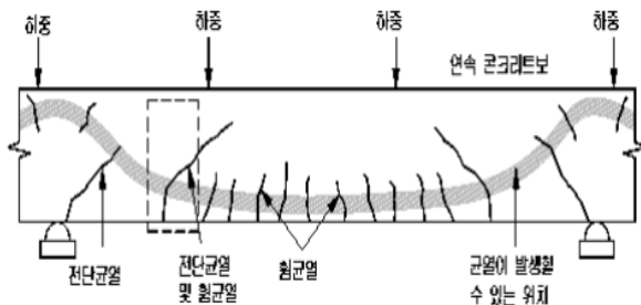
【그림 3.2.4】 콘크리트 거더에 발생하는 균열의 유형과 위치
