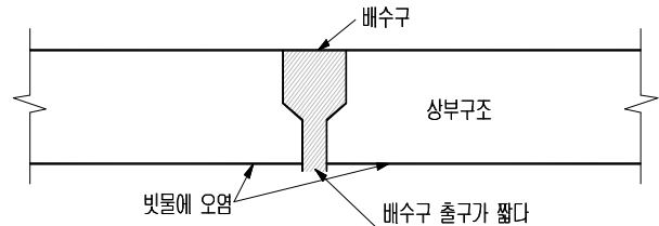
【그림 3.2.22】 배수구 길이 부족
