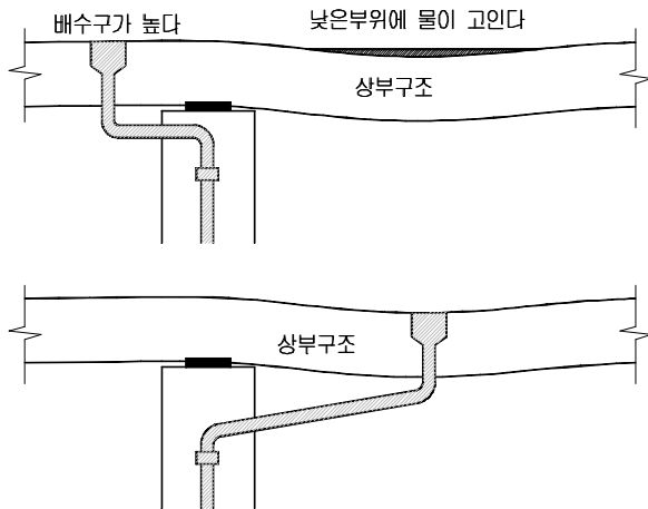
【그림 3.2.21】 배수구 물고임
