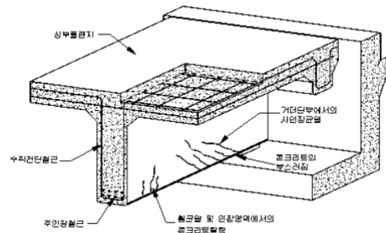
【그림 3.2.5】 철근콘크리트 거더의 조사부위
